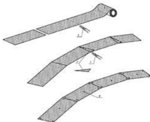
1 - инструмент; 2 - вырезанный клин сетки; 3 - анкеровка сетки
