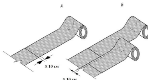
А - поперечный стык; В - продольный стык
